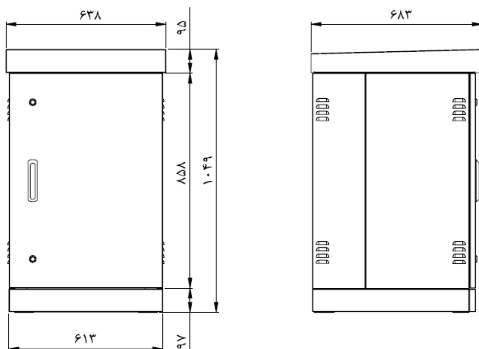
نقشه کابینتی نمونه به ارتفاع ۱۸ یونیت و عمق ۶۰ سانتیمتر
